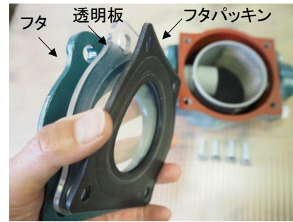
③フタを外す。フタ→透明板→パッキンの順になっています。
