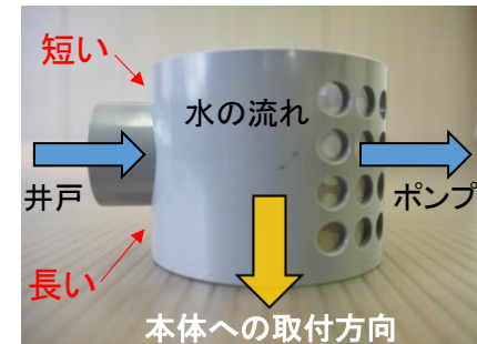
⑧ストレーナーは向きがあります。注意して取り付けてください。
