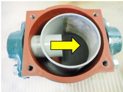
⑤ストレーナーを矢印の方向へずらす。
