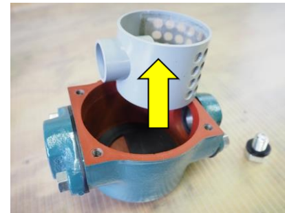
⑦ストレーナーと砂取器内部をたわし等で水洗いして下さい。
