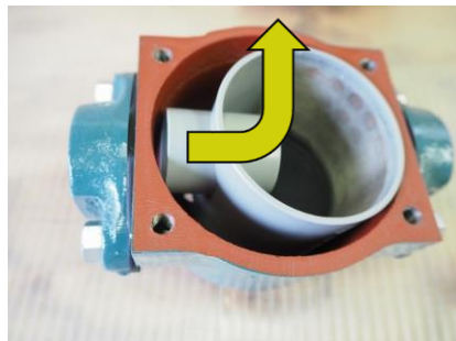
⑥下流方向に押しながら持ち上げるとストレーナーが外れます。
